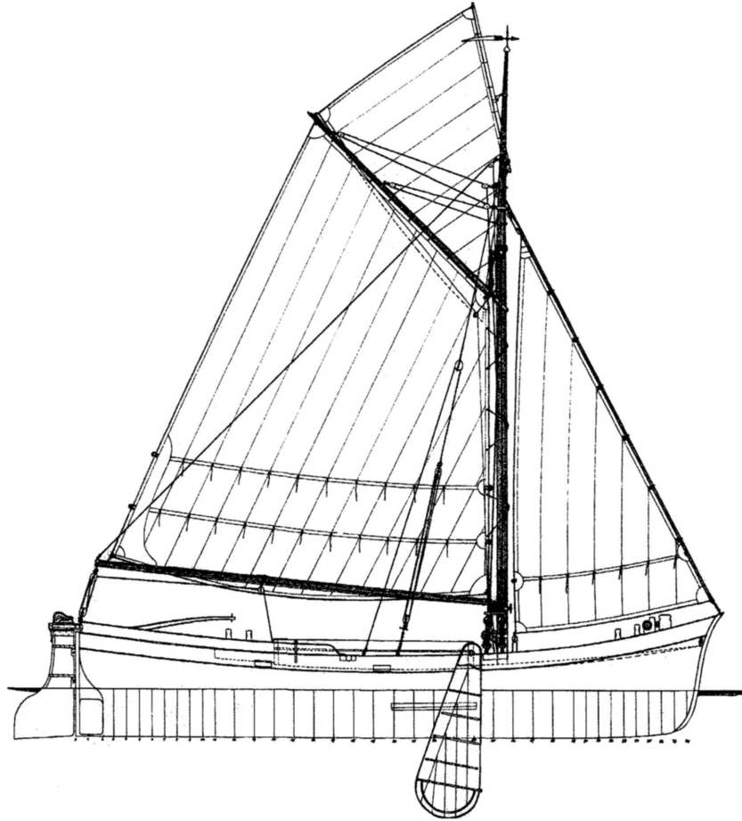
Schiffsriss von der ELFRIEDE
